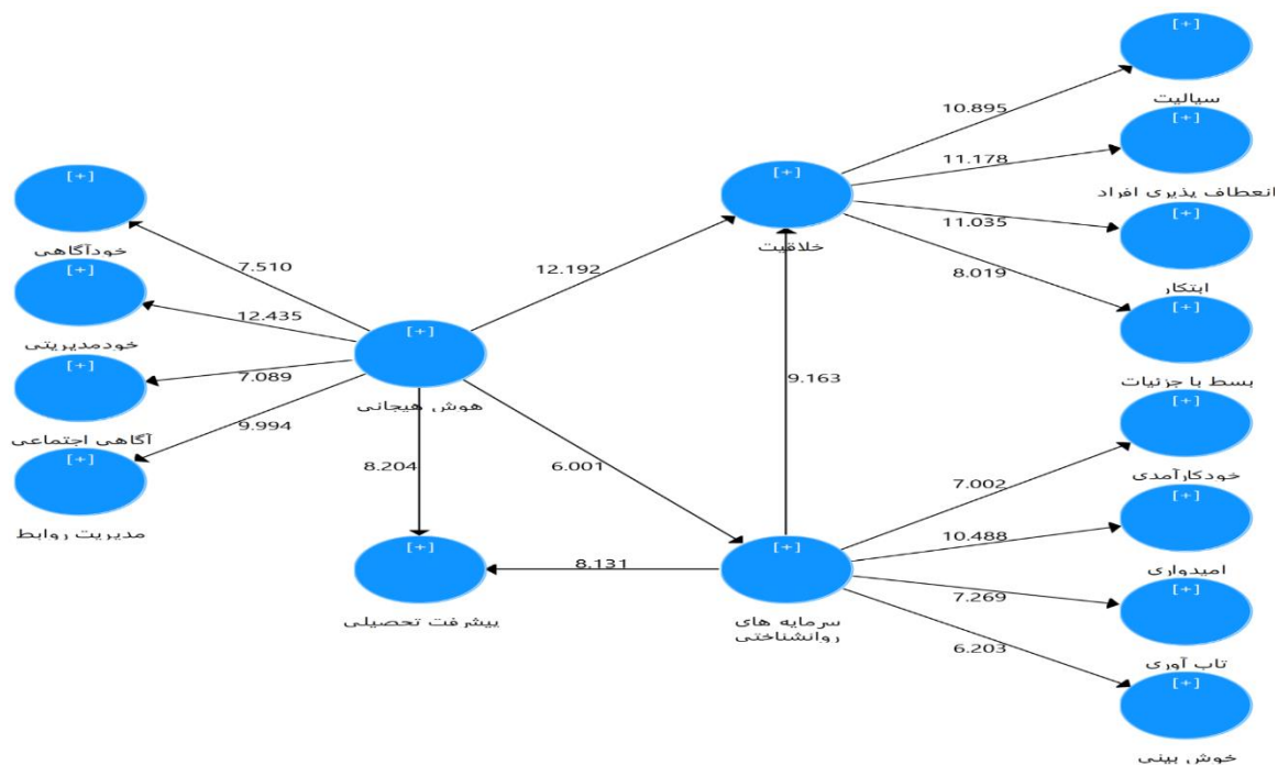
شکل ۱. ضرایب معناداری T-VALUE در مدل مفهومی
