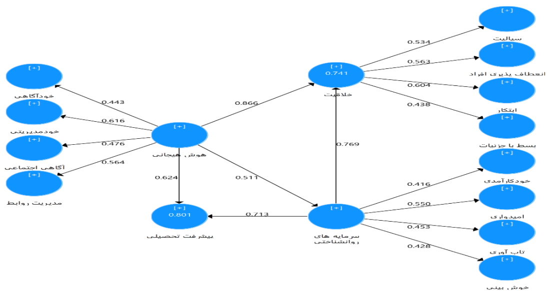
شکل ۲. ضریب مسیر در مدل مفهومی
