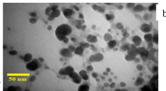
شکل ۱: تصاویر UV-vis (a) و TEM نانوذرات اکسید روی (b)
